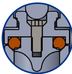
Conjunto de Vedação com Defletor para direcionamento de fluxo
